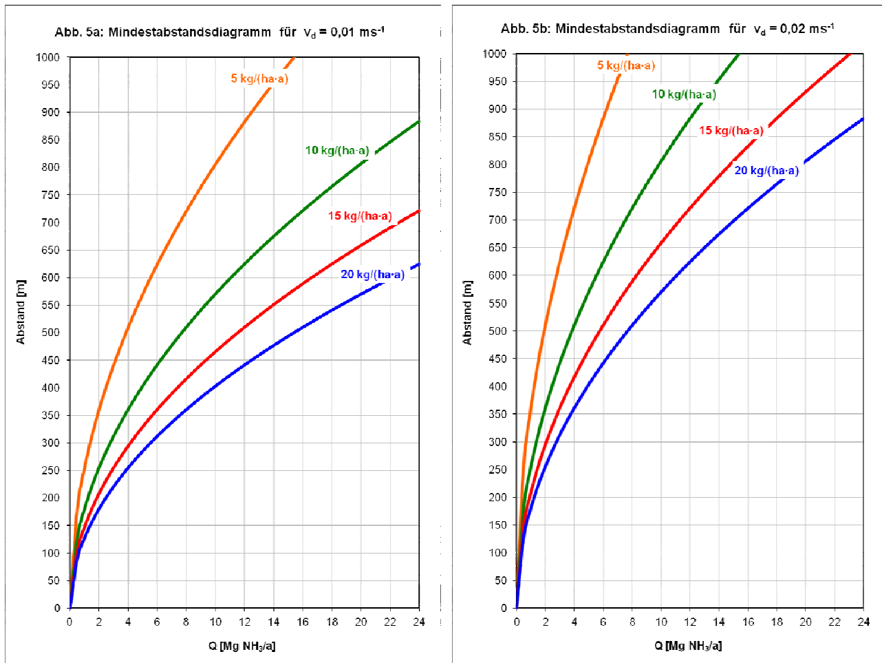
Abb. 5: Mindestabstandsdiagramm für Stickstoffdeposition für eine anlagenbezogene Zusatzbelastung von 5 \text{ kg ha}^{-1}\cdot\text{a}^{-1} , 10 \text{ kg ha}^{-1}\cdot\text{a}^{-1} , 15 \text{ kg ha}^{-1}\cdot\text{a}^{-1} und 20 \text{ kg ha}^{-1}\cdot\text{a}^{-1} mit v_d = 0,01 m/s (5a) und v_d = 0,02 m/s (5b).
