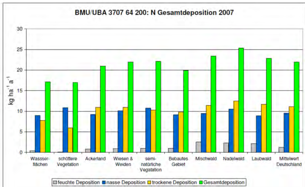
Abb. 4: Mittlere Stickstoffgesamtdeposition für das Jahr 2007 nach Depositionsflüssen und Landnutzungsclassen (Datenquelle: BMU/UBA 3707 64 200, Bultjes et al., 2011)
