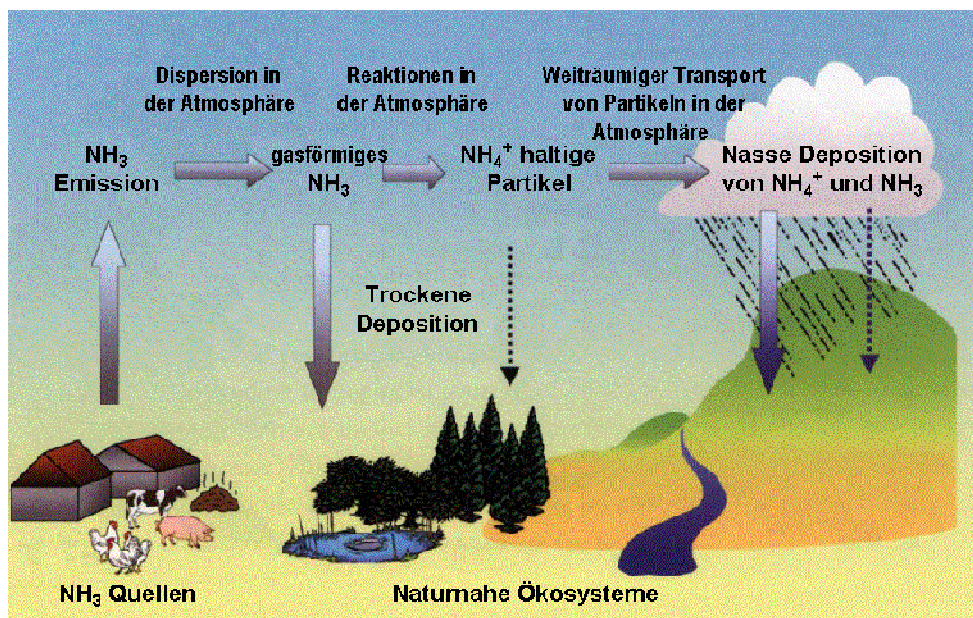
Abb. 2: Entstehung und Ablagerung von Ammoniak-/Ammoniumverbindungen (Quelle, abgeändert: Ammonia in the UK, DEFRA 2002)
