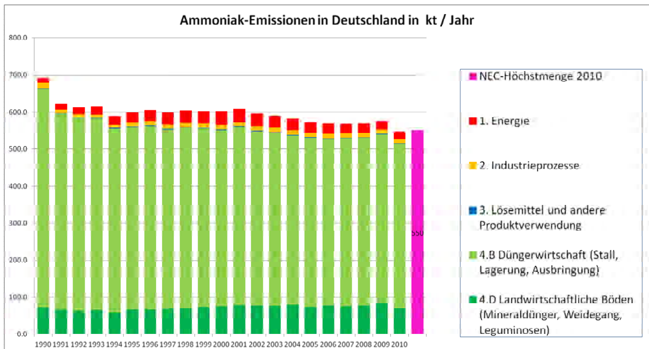
Abb. 1: Ammoniakemissionen nach Sektoren in Deutschland (Quelle: UBA [8])
