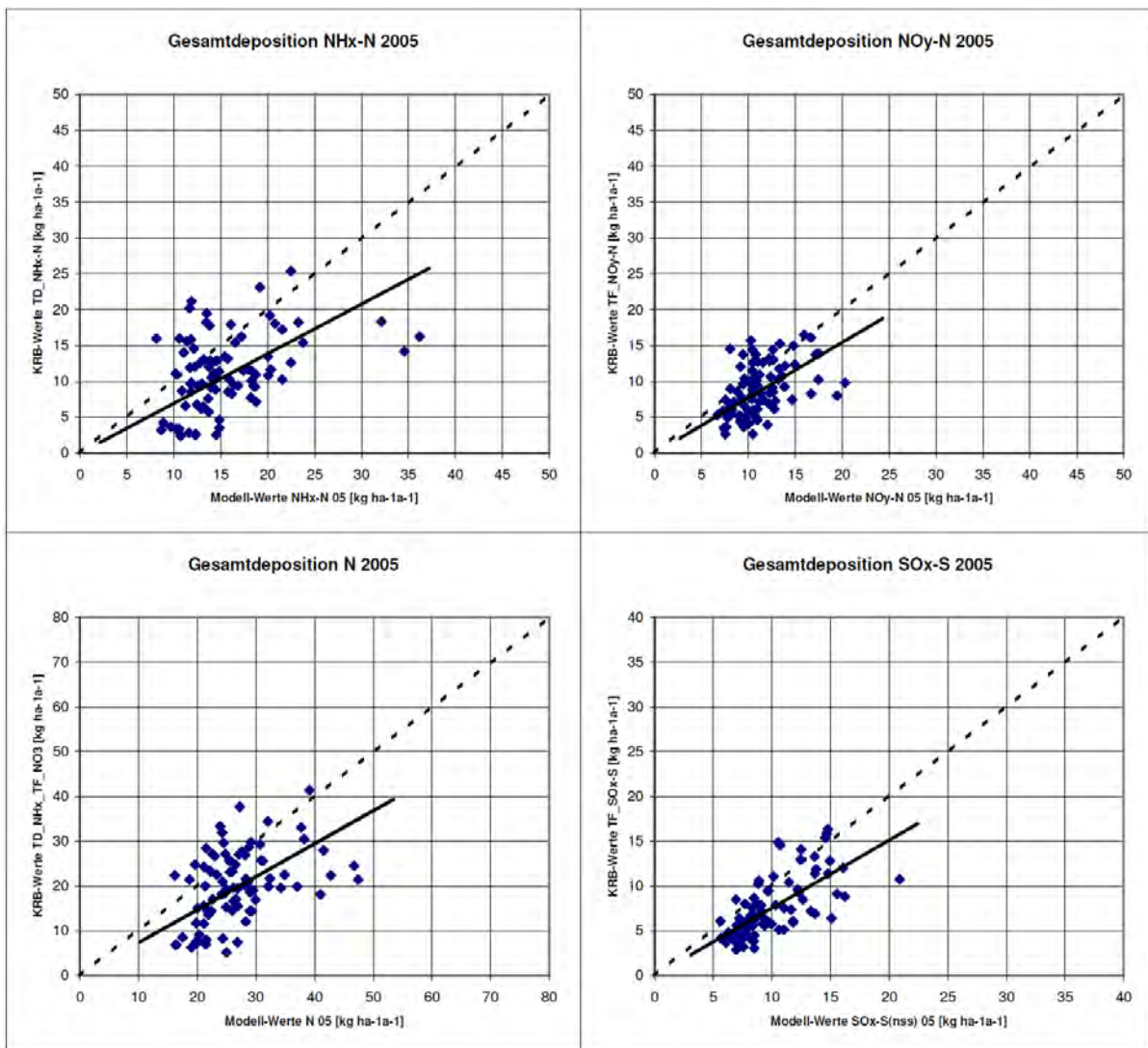
Abbildung A.I.5: Vergleich der Modell-Ergebnisse der flächenhaften Kartierung der Gesamt-Deposition für \text{NH}_x\text{-N} , \text{NO}_y\text{-N} , N und \text{SO}_x\text{-S} 2005 mit Schätzungen der Gesamt-Deposition aus Kronenraumbilanz-Berechnungen (Quelle: Gauger, 2011 [30a])
