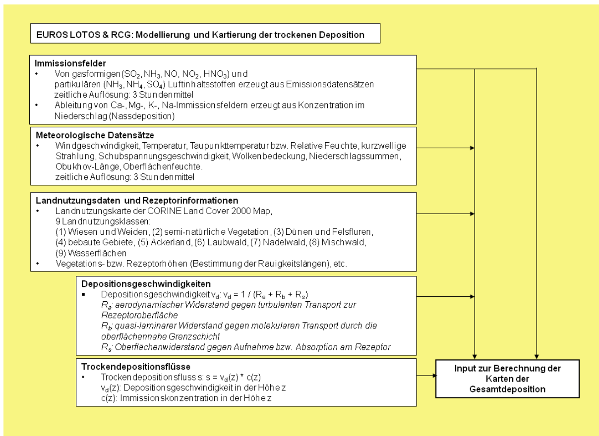
Abb. A.1.3: Eingangsdaten und generelle Abfolge der Modellberechnung der trockenen Deposition
