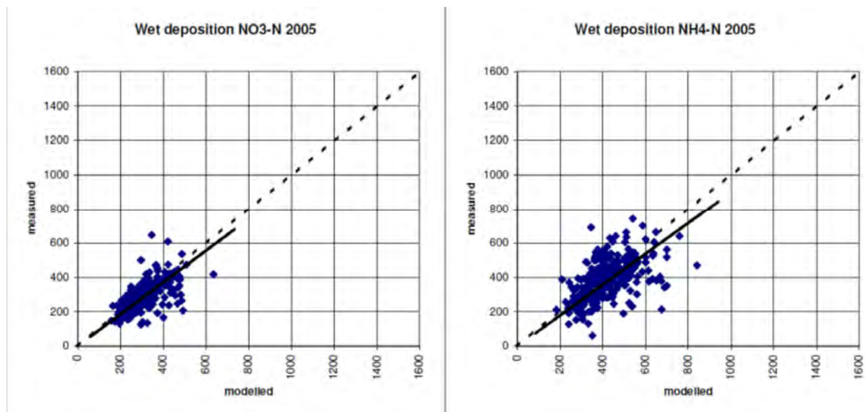
Abb. A.I.2: Vergleich von Karten- und Messwerten der nassen Depositionsfrachten von Ammoniumstickstoff und Nitratstickstoff im Jahr 2005 [ \text{eq ha}^{-1} \text{a}^{-1} ]
